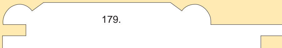
Kragerøkledning. Forside: ru 21 x 120 mm
