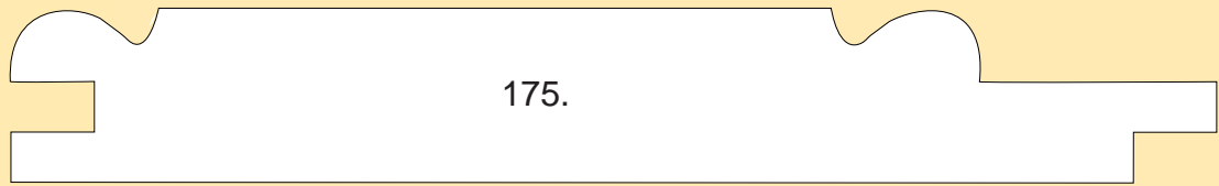
Sveitzerkledning. Forside: ru eller glatt 21 x 120 / 145 mm
